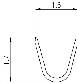
A-A SECTION
